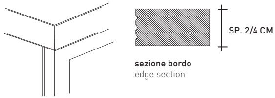
Bordo ABS Spessore 2 cm ABS edge Thickness 2 cm
